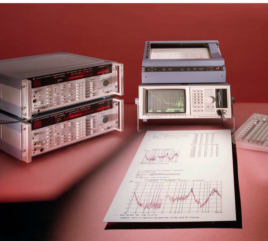
Bild 10: Messempfänger ESH3 (9 kHz bis 30 MHz, oben) und ESVP (20 bis 1300 MHz) mit Spektrum-Monitor EZM.
