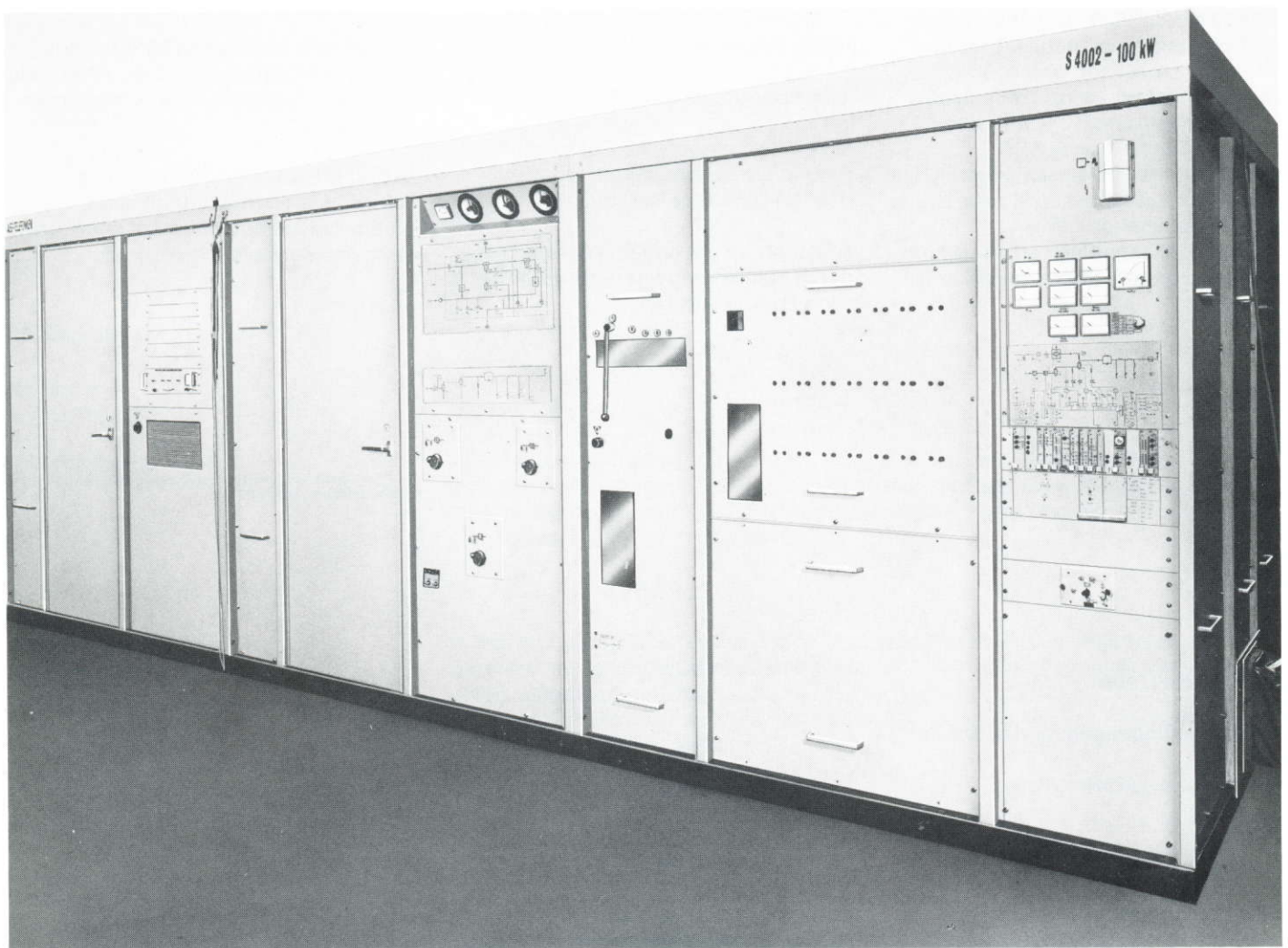
Bild 1: 100-kW-MW-Rundfunksender S 4002
