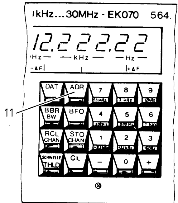
Bild 2.42 Adressenschalter
