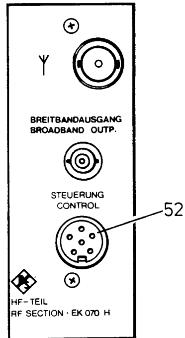
Bild 2.23 Steueranschluß
