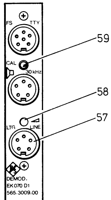
Bild 2.24 Leitungsausgänge
