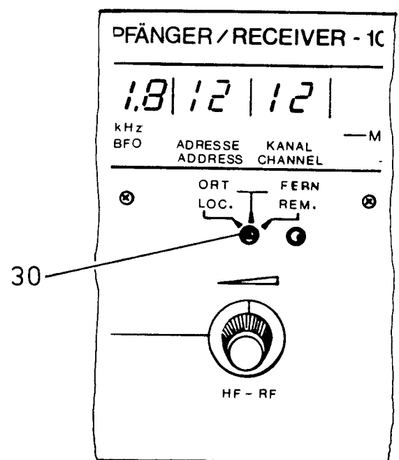
Bild 2.43 Ort/Fern-Schalter
