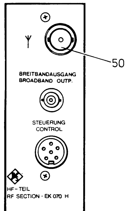
Bild 2.22 Antennenbuchse
