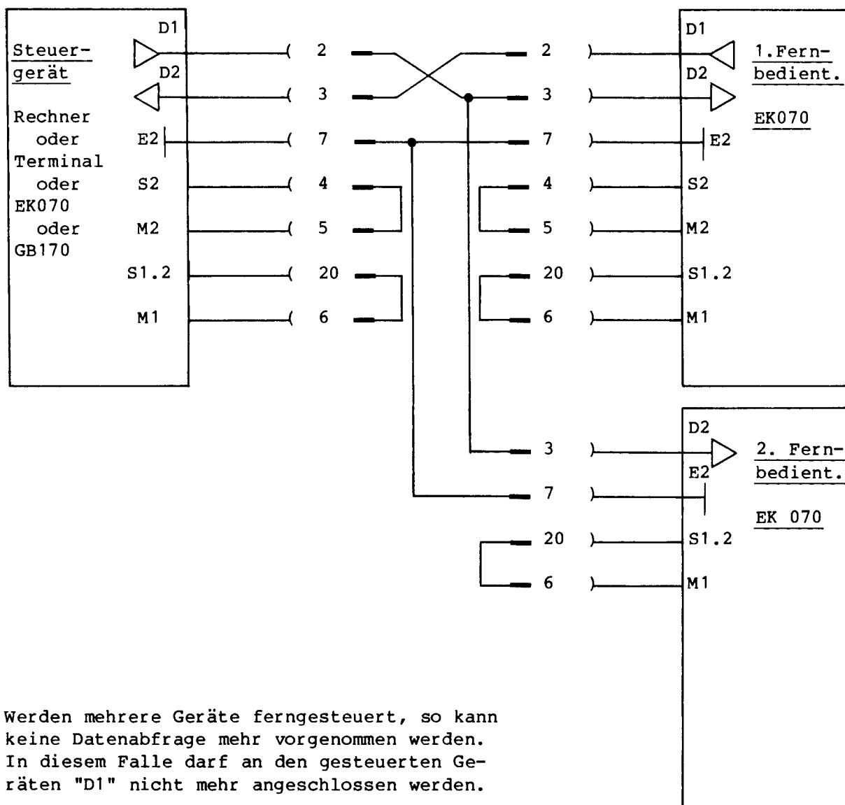
Bild 2.33 Zusammenschaltung nach V.24/V.28-Norm
