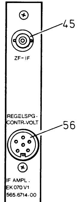
Bild 2.27 Regelspannungsausgang
