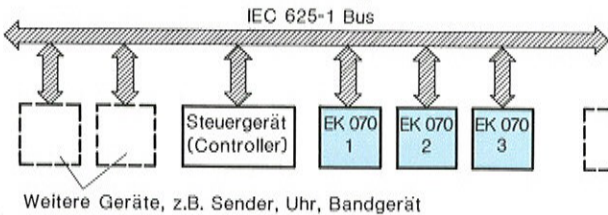
Fernsteuerung und Abfrage über IEC-Bus
