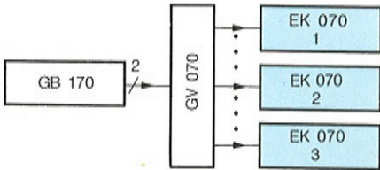
Fernsteuerung mehrerer Empfänger durch das Bediengerät GB 170
