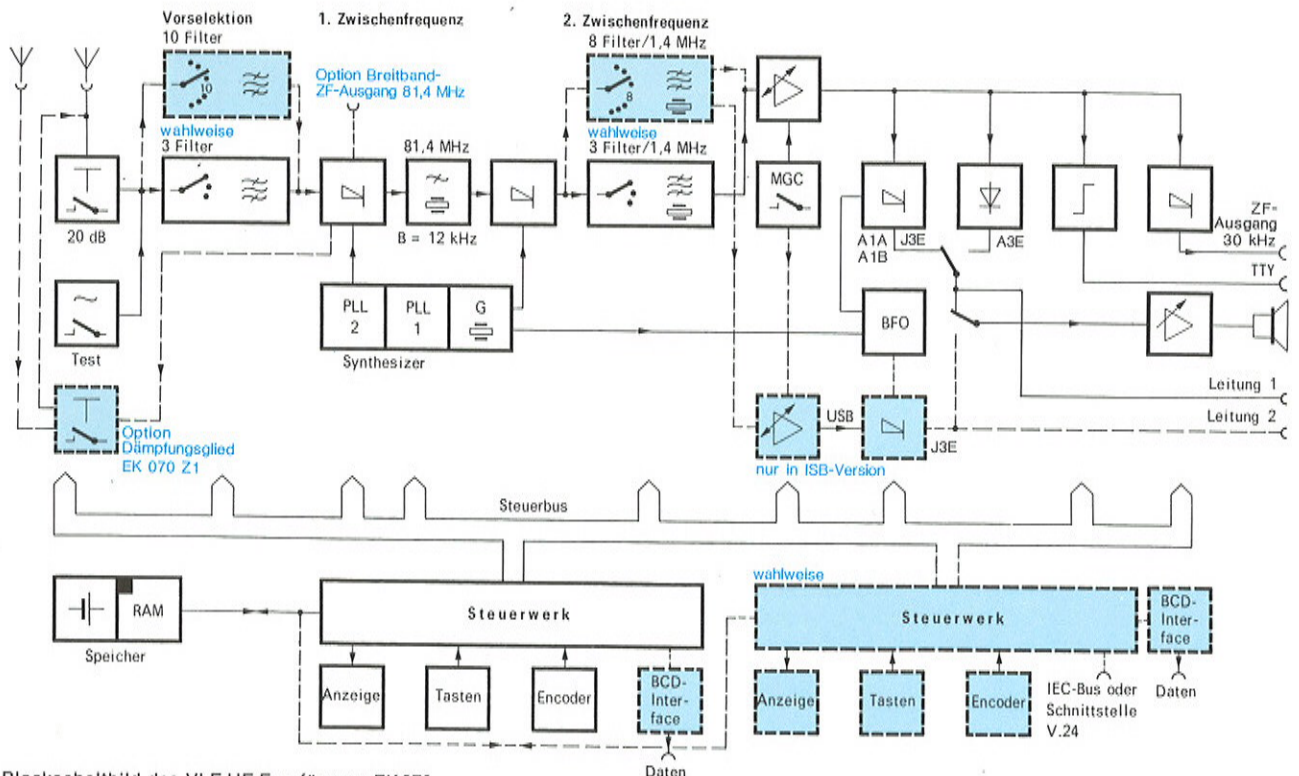
Blockschaltbild des VLF-HF-Empfängers EK070
